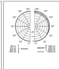
Polardiagramm
