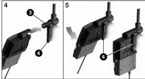
Fig. 3: Fixar o adaptador com o emissor de bolso no cone do microfone
