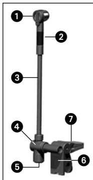
Fig. 1: Microfone C 519 M/C 519 ML
